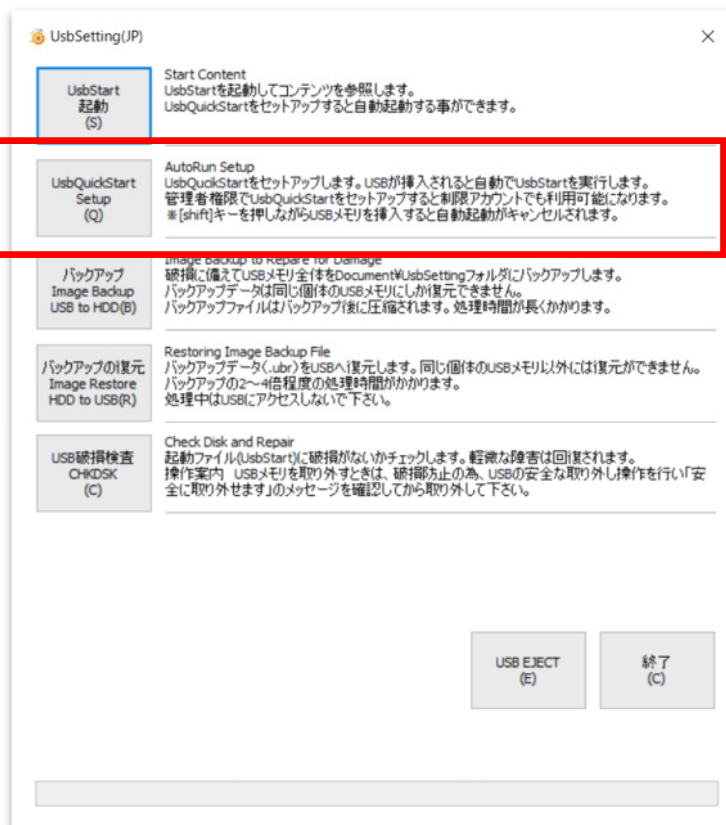
UsbSetting.exe
